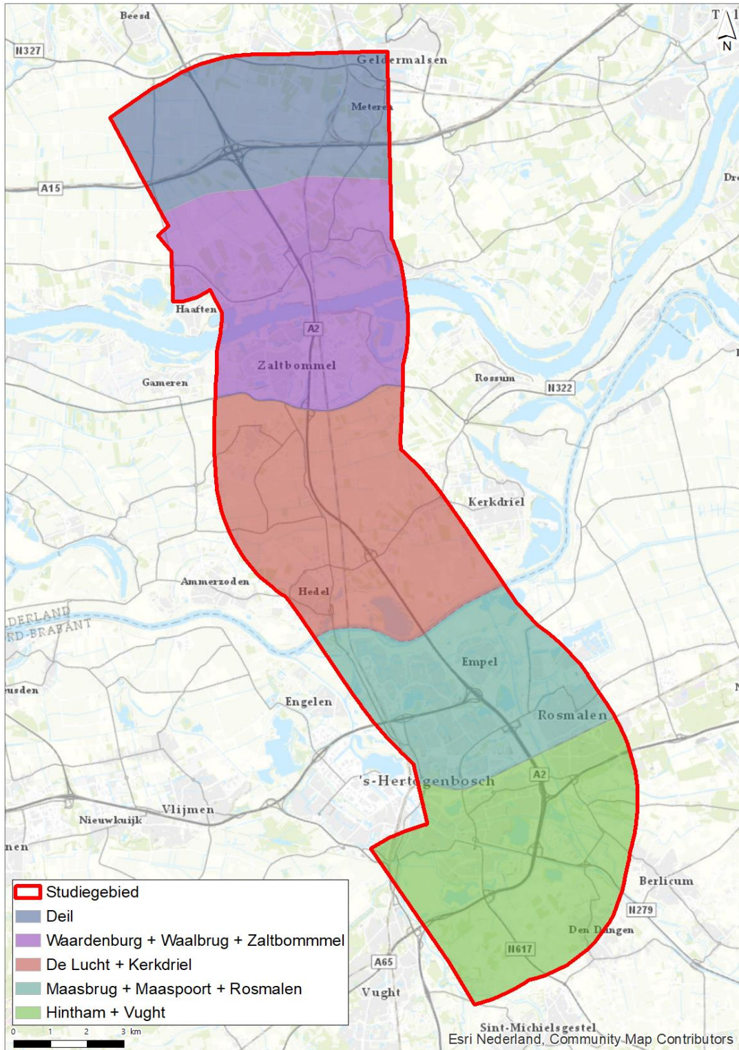
Afbeelding 4.1 Studiegebied
