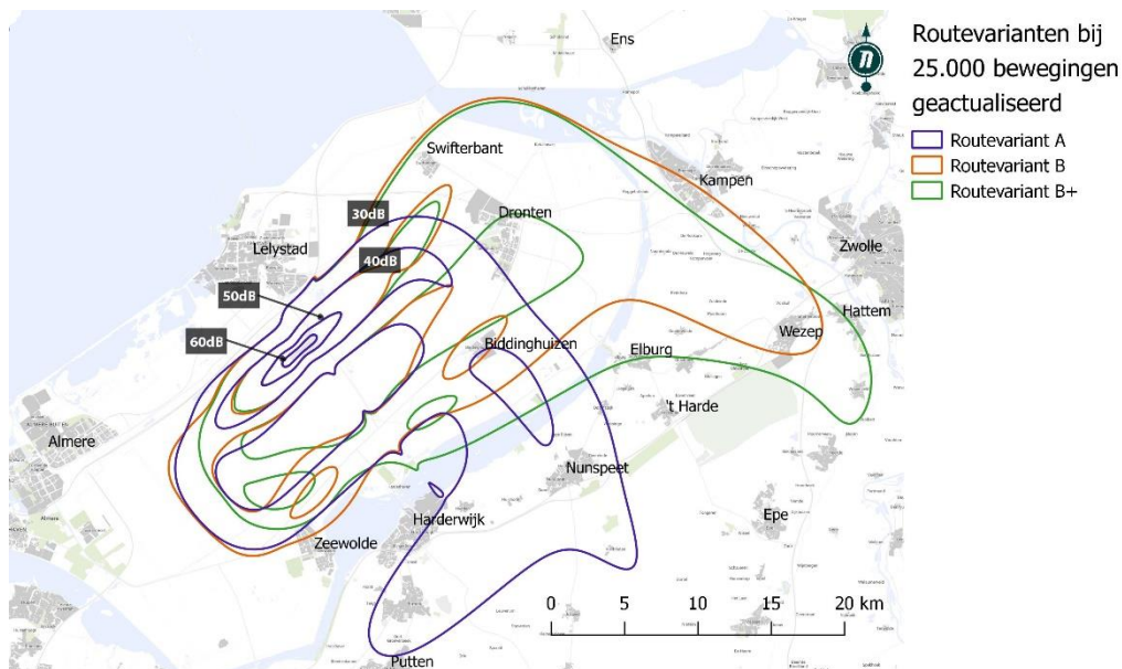
Figuur 24 – Vergelijking van de geactualiseerde 30 t/m 60 L_{night} contouren bij 25.000 bewegingen.
