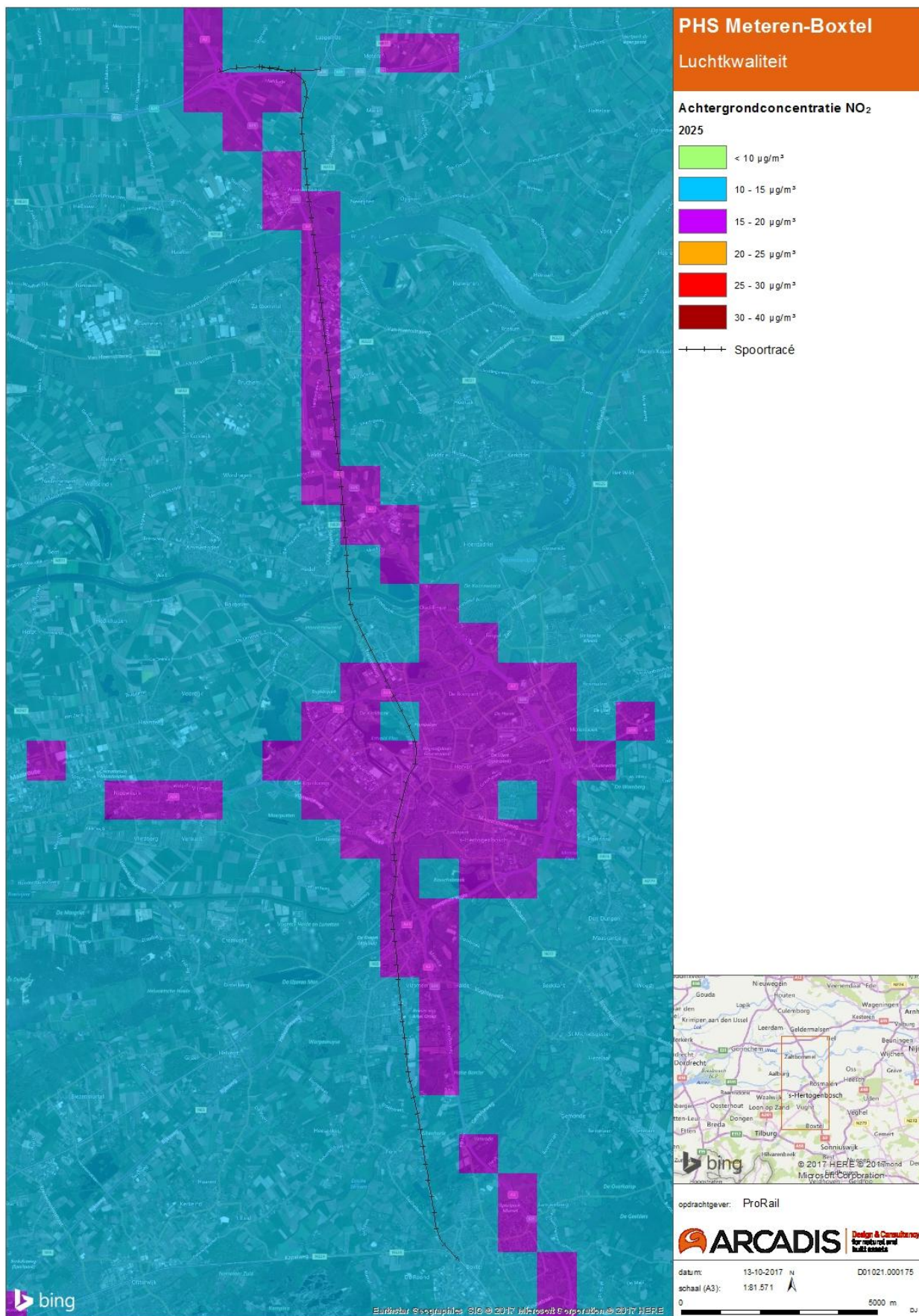
Afbeelding 28: Achtergrondconcentratie NO 2 , 2025
