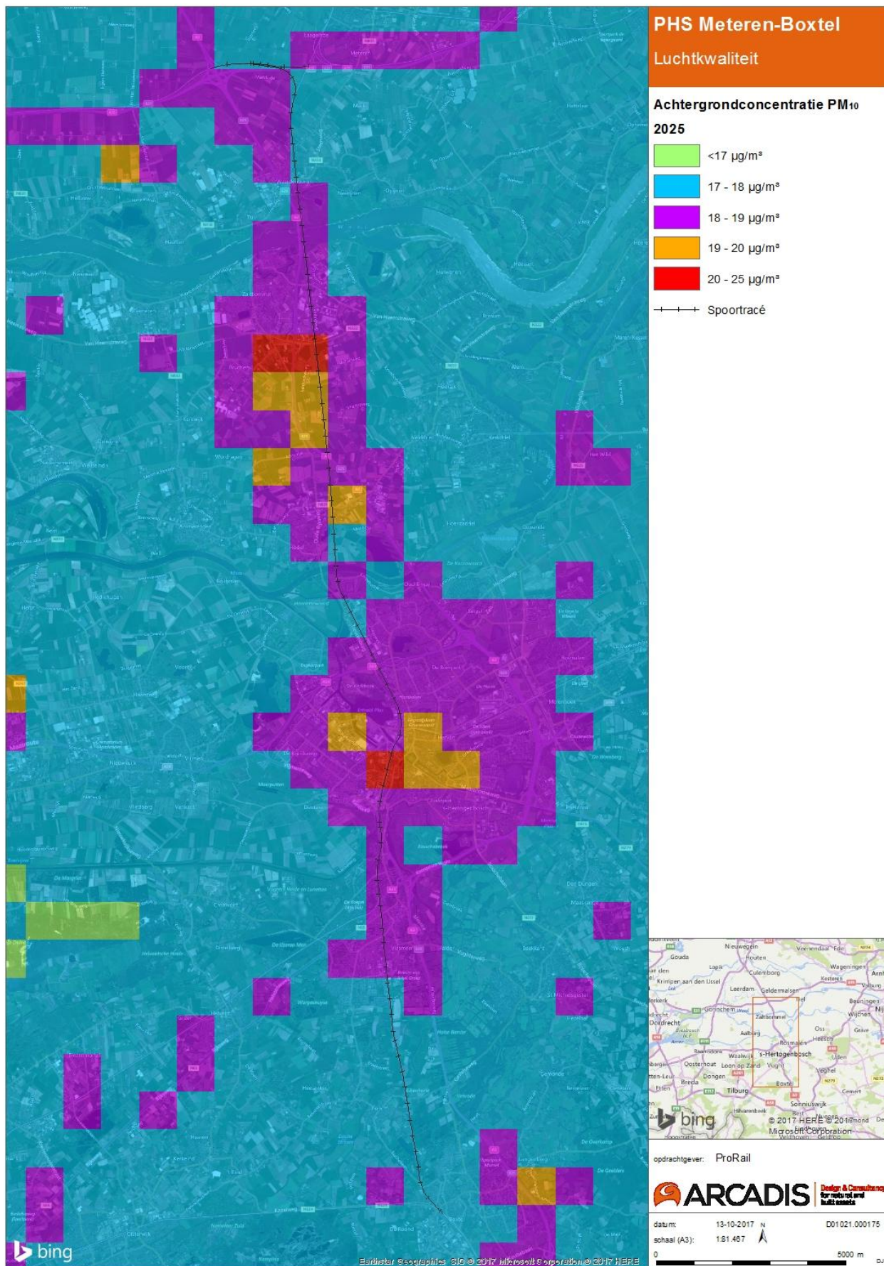
Afbeelding 29: Achtergrondconcentratie PM 10 , 2025
