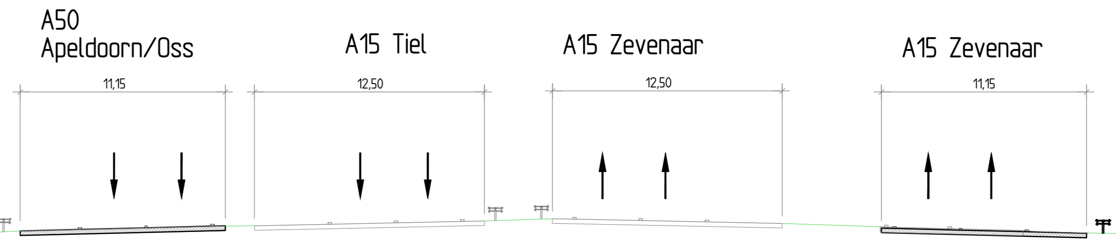
Dwarsprofiel 2-2 Metrening A15 155760 Schaal 1:200
