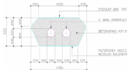
GRINDKOFFER MET 2 DRAINS
