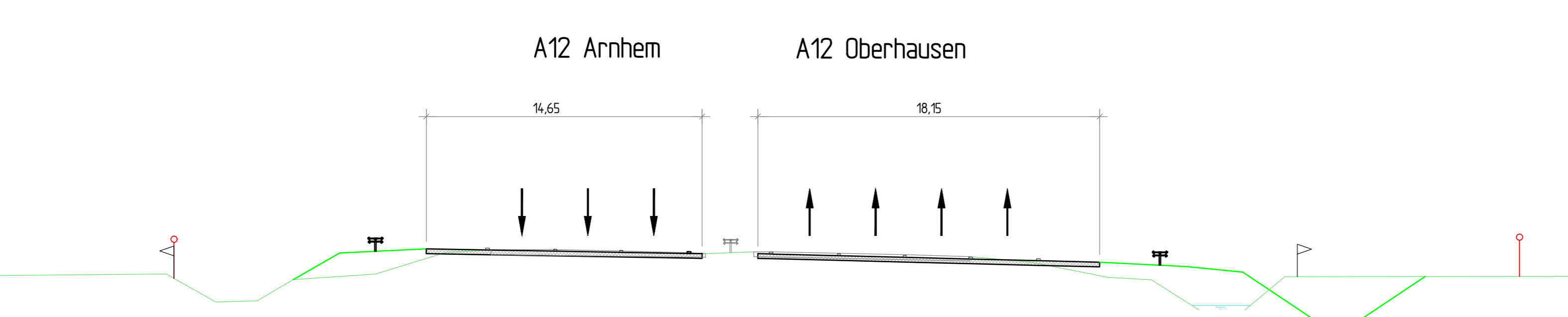
Dwarsprofiel 24-24 t.o.v. as A12 Metrening A12 141850 Schaal 1:200
