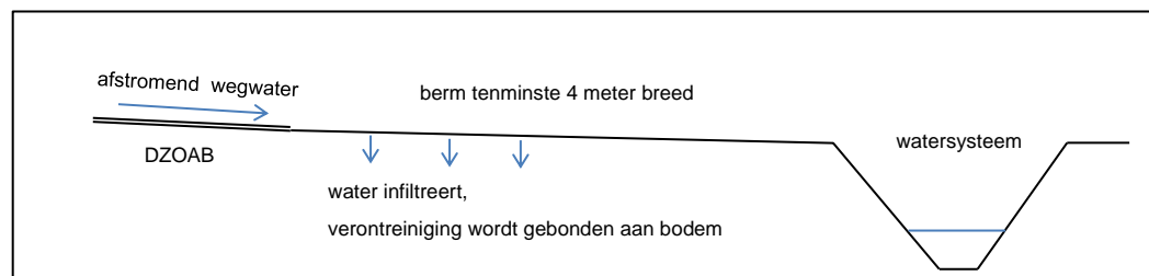
Figuur 4.1 Principeprofiel lozen op of in de bodem bij een berm van tenminste 4 meter
