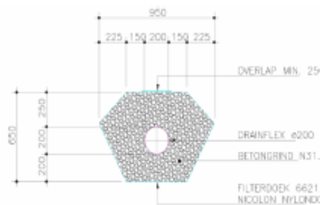
GRINDKOFFER MET 1 DRAIN
