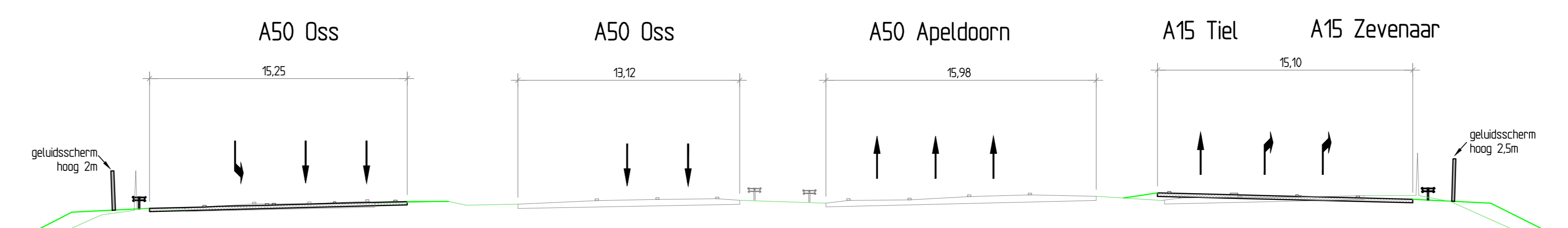
Dwarsprofiel 1-1 Metrening A50 154250 Schaal 1:200
