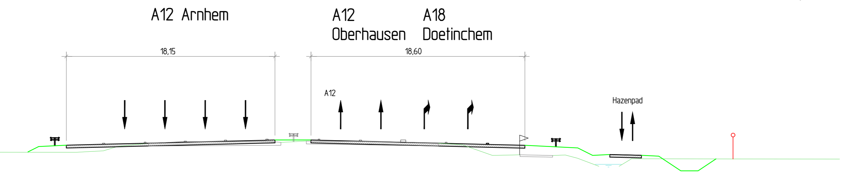
Dwarsprofiel 27-27 t.o.v. as A12 Metheuring A12 146750 Schaal 1:200
