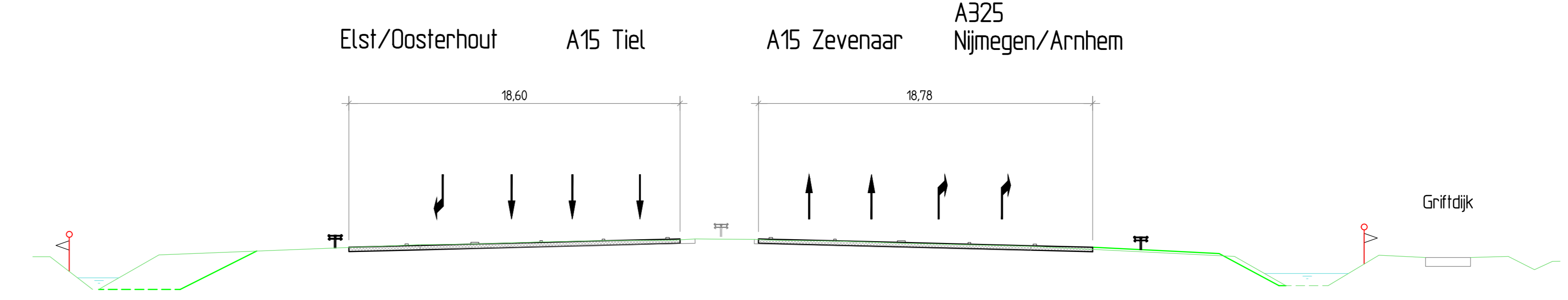
Dwarsprofiel 6-6 Methrening A15 160600 Schaal 1:200
