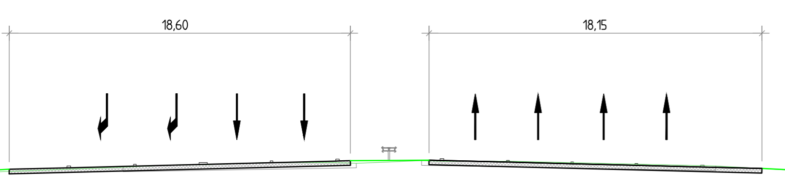
Dwarsprofiel 3-3 Metrening A15 156345 Schaal 1:200
