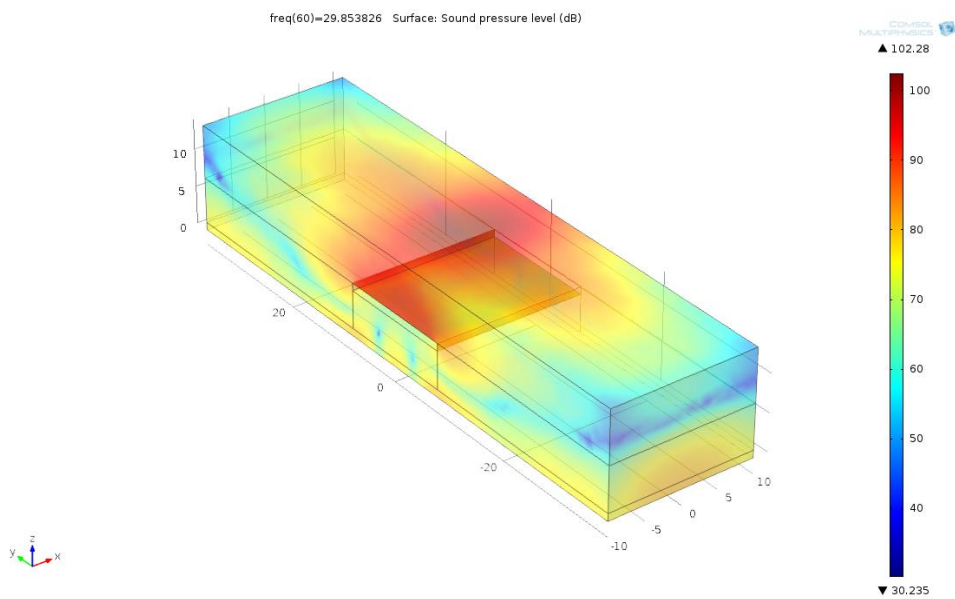
Figuur 4: Als Figuur 1, waarbij de onderkant van het brugdek van resonatoren is voorzien.
