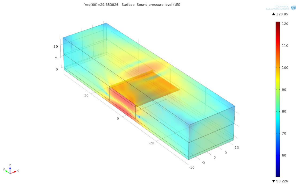
Figuur 3: Als Figuur 1, waarbij twee wanden onder de brug van resonatoren zijn voorzien.
