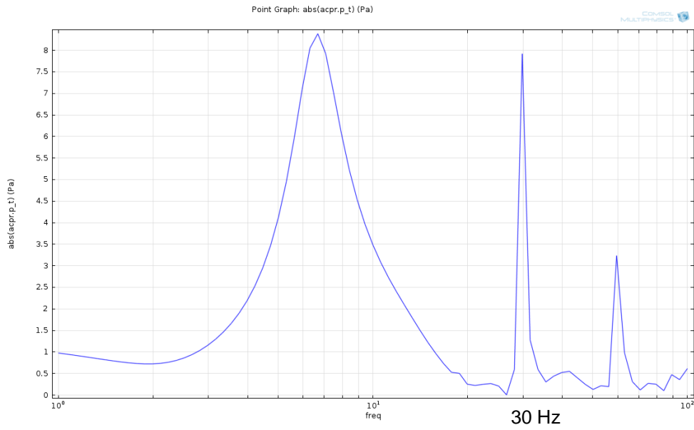
Figuur 5: Spectrum van de geluiddruk aan de zijkant van de brug, links in Figuur 1.
