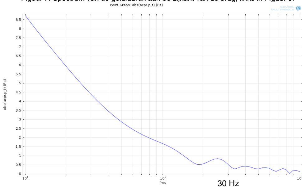
Figuur 8: Spectrum van de geluiddruk aan de zijkant van de brug, links in Figuur 4.
