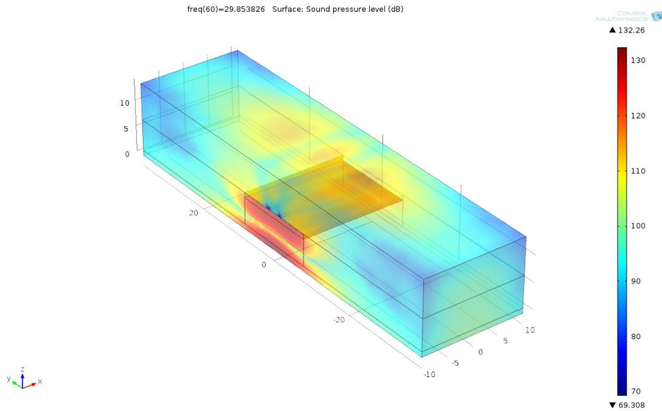
Figuur 1: Resultaat van een eenvoudig eindig elementen model van de brug met brugdek, kade, wateroppervlak, en omgeving; geluiddruk bij een homogene verticale beweging van het brugdek met een versnelling van 1 \text{ m/s}^2 bij een frequentie van 29,85 Hz, zonder resonatoren op de wanden onder de brug en de onderkant van de brug.
