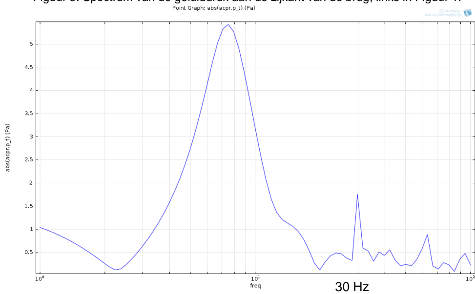
Figuur 6: Spectrum van de geluiddruk aan de zijkant van de brug, links in Figuur 2.
